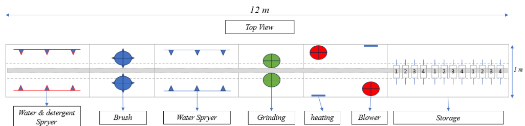
Gambar 4. PRO GALO Tampak Atas
